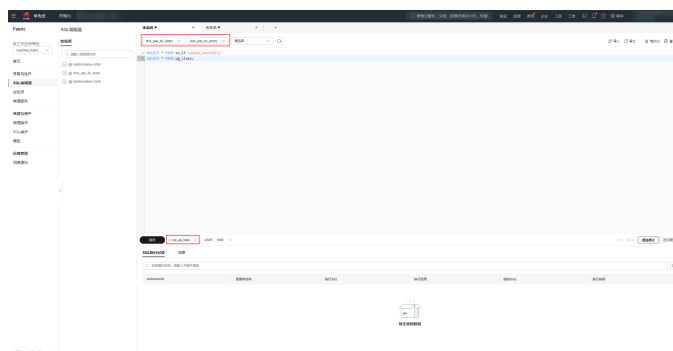
图 3-2 运行 SQL
